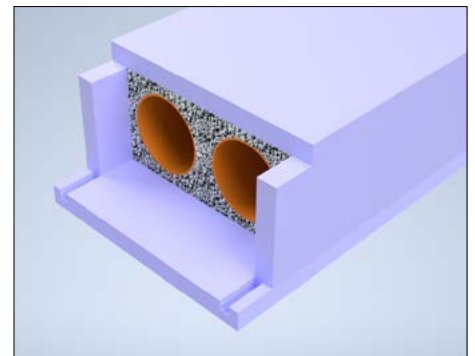
Kassene leveres i tykkelse 50mm og 100mm avhengig av isolasjonsbehov.
